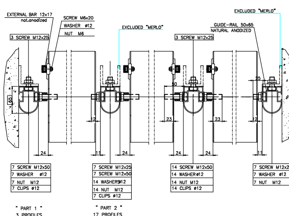
Vista in pianta: Frangisole orizzontale con telai tipo E
