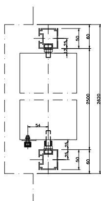
Vista in sezione: Frangisole verticale con telai tipo D
